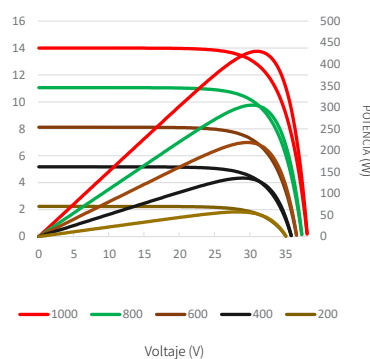
Curvas de corriente-voltaje y potencia-voltaje (430W)
